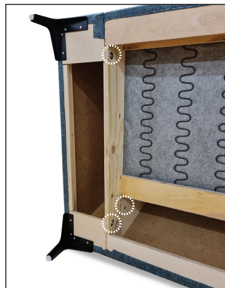
Kuva 2. 3 kpl pultti
